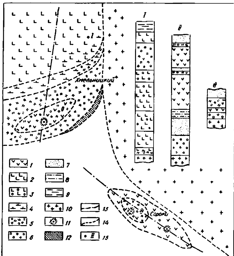
Рис. 25. Сопоставление геологических разрезов терригенно-вулканогенной формации Подолии и положение в них пирокластических пород:
