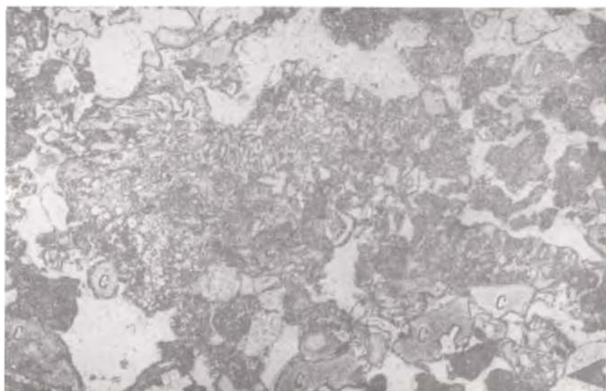
Рис. 22. Туф средне-крупнообломочный. Лапиллы витрофировых базальтов (черные) и сапонитизированных тонкопузыристых стекол (с) цементированы цеолитами. Видна тонкая лимонитовая кайма, оконтуривающая обломки стекол. Пикколи \bar{\bar{}} , \times 50 , скв. 14-СП, глуб. 253,2 м.
