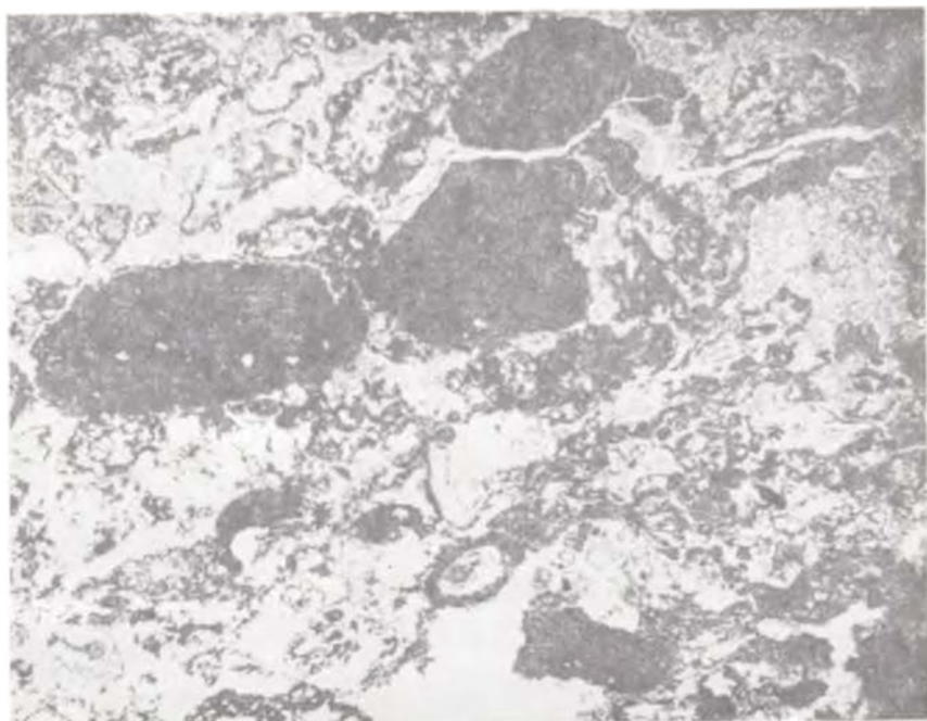
Рис. 28. Туф псефитовый, витрокластический. Николаи П., \times 30 .
