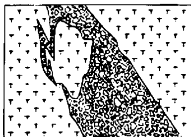
Рис. 13. Эксплозивная брекчиевая дайка с апофизами. Береговское месторождение. Штольня 1, расщелка 13, правая стенка:
