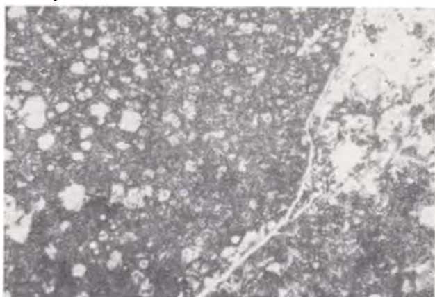
Рис. 46. Кластолава с обломками нефелинита (скв. Белоцерковская-232). Николи ||, \times 50 .
