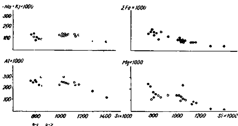
Рис. 31. Диаграмма распределения основных породообразующих элементов (атомные количества \times 1000 ):
