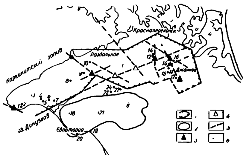
Рис. 40. Схема расположения центров мелового вулканизма в Равнинном Крыму, по Л. Г. Плахотному, М. Я. Апостоловой, В. Г. Бондаренко и В. А. Гордиевич (1971):
