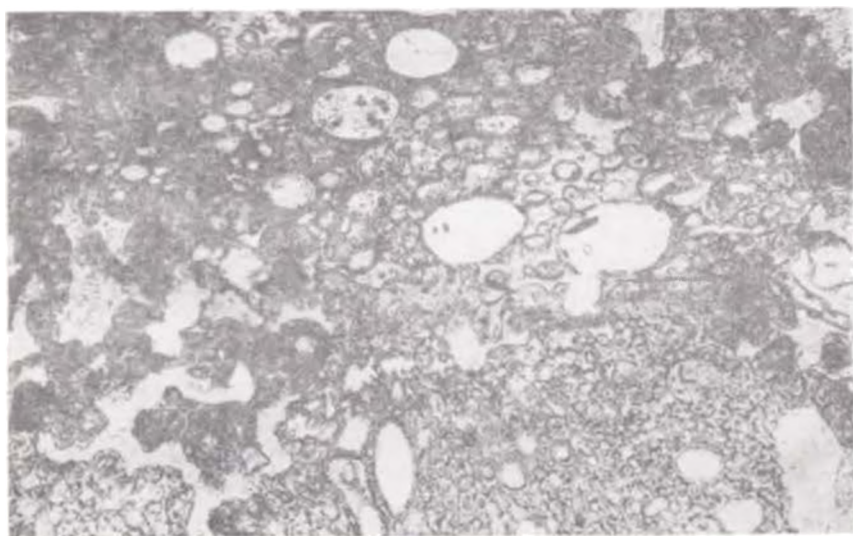
Рис. 19. Обломок желтовато-зеленого стекла из крупнообломочного туфа. Видны многочисленные округлые и овальные «пузыри», выполненные цеолитами. По периферии «пузыри» имеют слабодвупреломляющую радиальную каемку. Николь \parallel , \times 50 , скв. 15-СП, глуб. 576,0 м.
