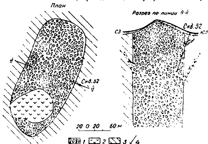
Рис. 11. Жерловина, выполненная брекчией и штоком андезито-базальта. Оленевский район:
