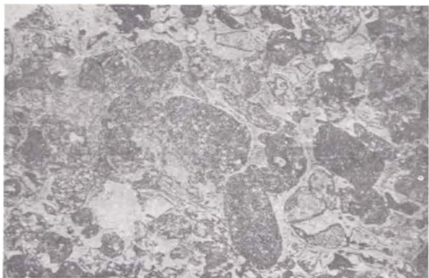
Рис. 29. Серповидные и неправильной формы выделения вулканического стекла. Николл \parallel , \times 30 .
