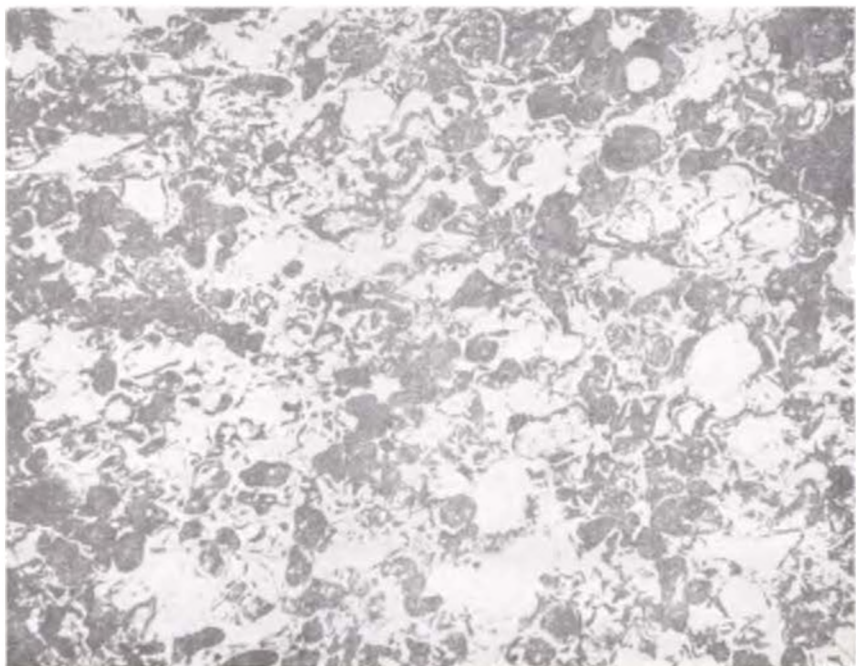
Рис. 27. Туф алевропсаммитовый, литовитрокластический. Микроскоп, \times 30 .
