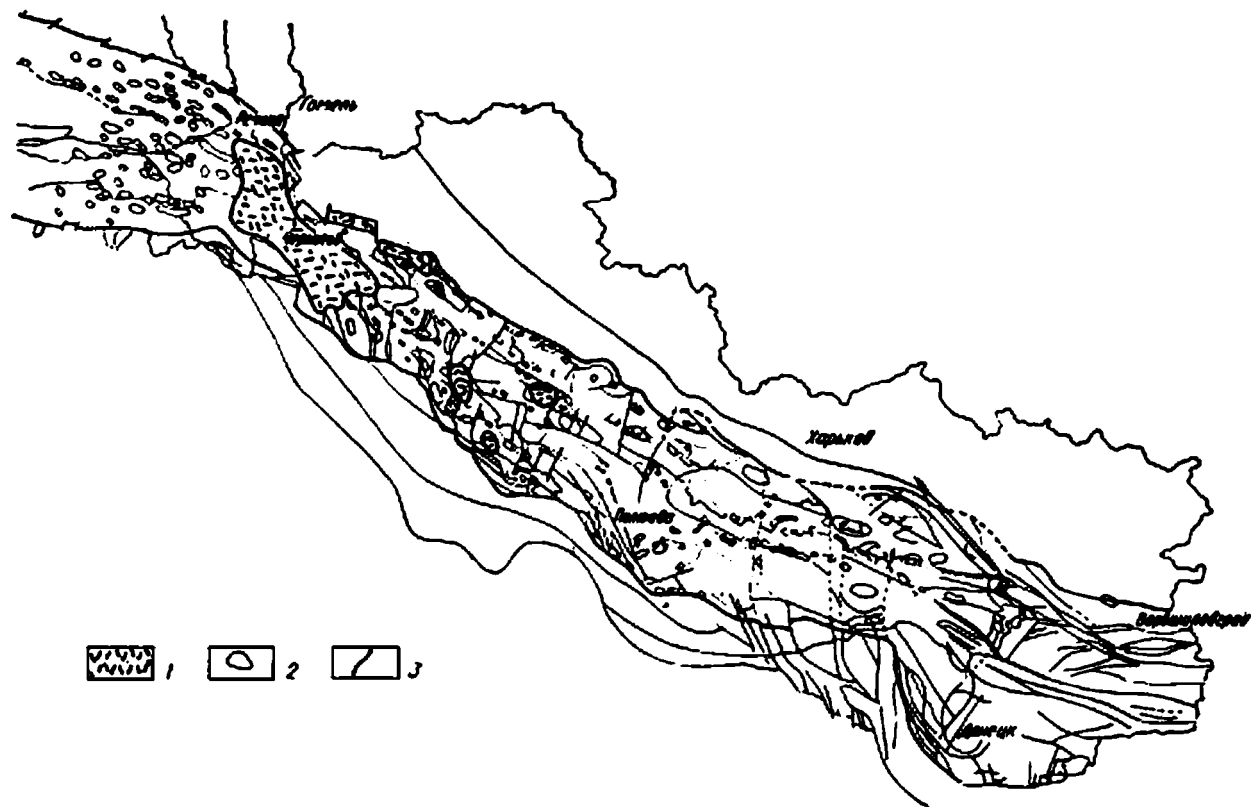
Рис. 43. Схема распространения девонской (D 3 fm) верхней вулканогенной толщи: 1 — вулканогенная толща; 2 — структуры осадочного чехла; 3 — глубокие разломы.
