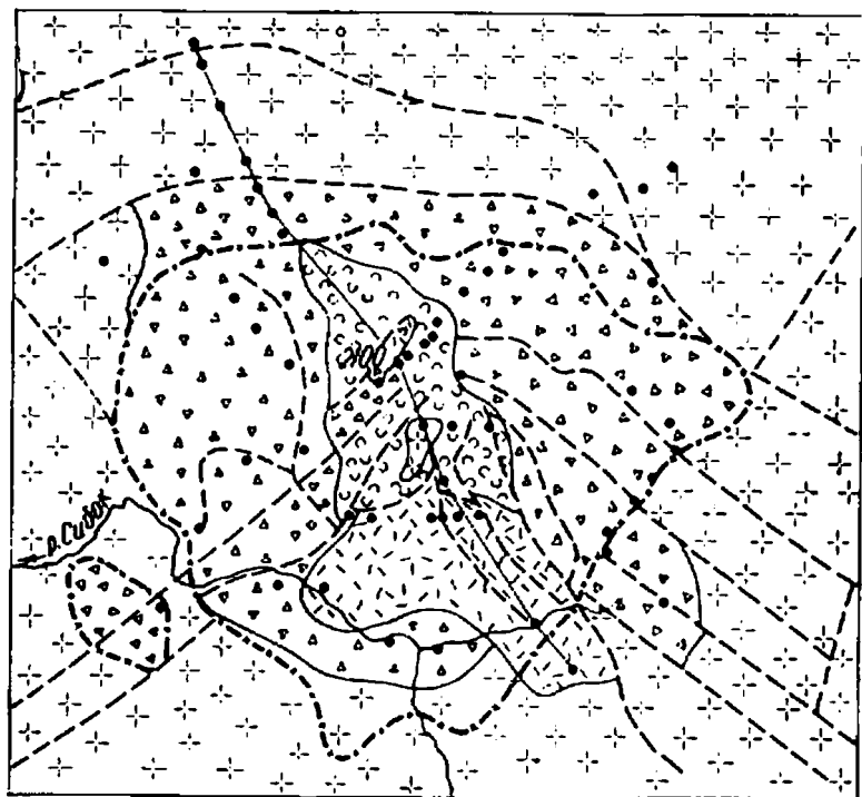
Рис. 50. Геолого-структурная карта Ильинского палеовулкана (составила С. С. Быстрельская с использованием материалов Г. А. Земскова (1968), Г. Г. Виноградова и данных детальных геофизических и буровых работ): 1 — лавобрекчии (жерловые образования); 2 — агломеративные лито- и кристаллоластические туфы; 3 — лавы трахиандезитового и трахиандезитового состава (покрышки); 4 — туфогенные гравелиты и вулканомиктовые конгломераты («туфобрекчии»); 5 — гранитоиды, мигматиты фундамента; 6 — граница кровли горизонта бесконечного электрического сопротивления, по данным ВЭЗ; 7 — радиальные и кольцевые разломы в пределах вулканической структуры по геологическим и геофизическим данным; 8 — скважины поисково-картировочного бурения и глубокие скважины.
