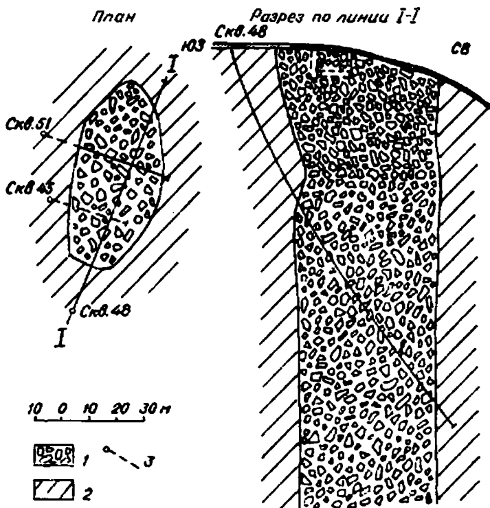
Рис. 10. Вулканическая жерловина, выполненная брекчией. Оленевский район.
