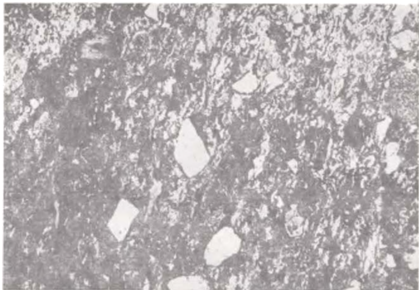
Рис. 32. Туф, обогащенный гидроокислами железа. Николь \parallel , \times 30 .
