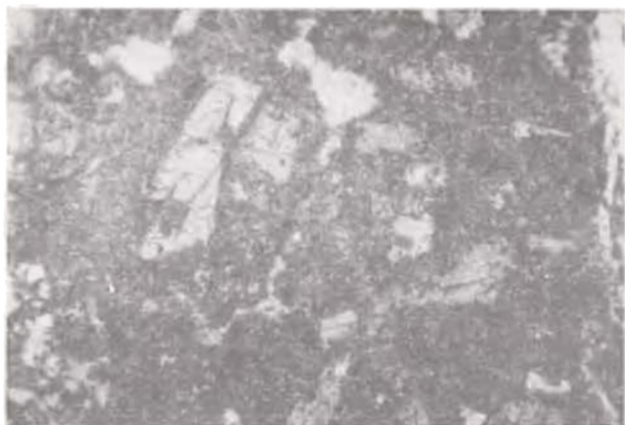
Рис. 44. Обломочный пироксен в базальтовом туфе (скав. Брусилов-2). Николи \perp , \times 100 .
