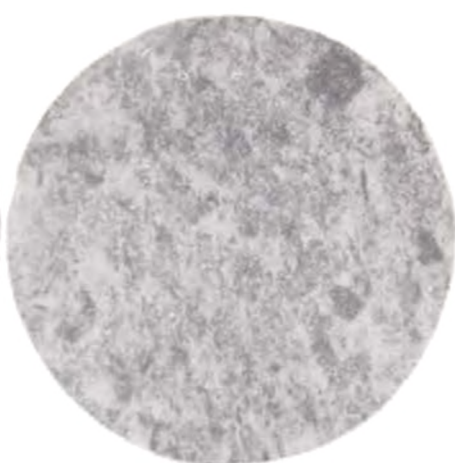
Рис. 4. Туффит. Верхнеменилитовая подсвита, р. Чечва. Без анализатора, \times 100 .
