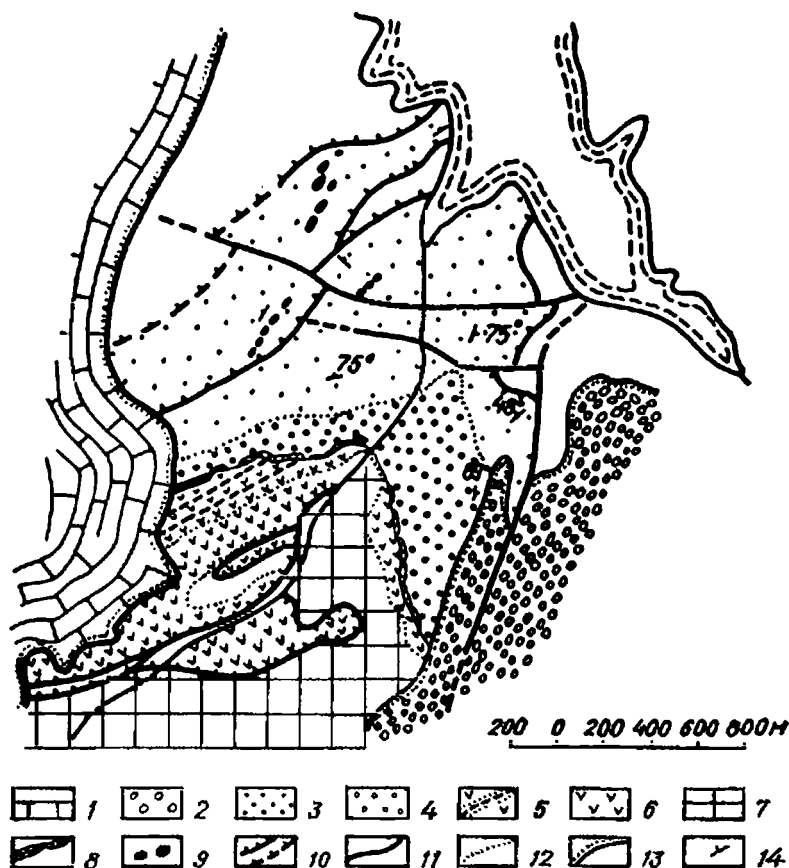
Рис. 34. Схематическая геологическая карта района сел Лозовое — Ук-раинка, по А. И. Шалимову:
