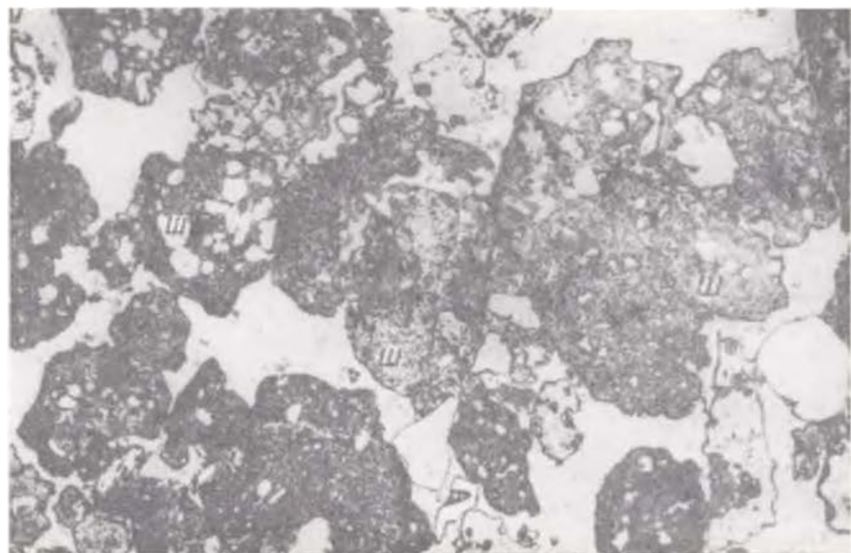
Рис. 20. Туф базальтовый среднеобломочный. Основная масса обломков представлена тонкопузыристыми шлаками (ш) и глалобазальтами. Цемент анальцимовый порового типа. Пикולי ||, > 50, скв. 1-СП, глуб. 454,2 м.
