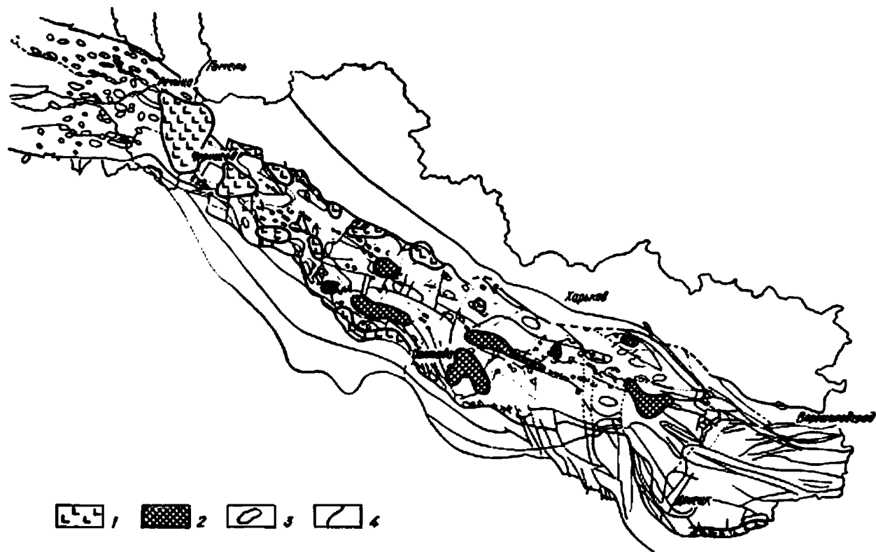
Рис. 42. Схема распространения девонской ( D_3,lg ) нижней вулканогенной толщи
