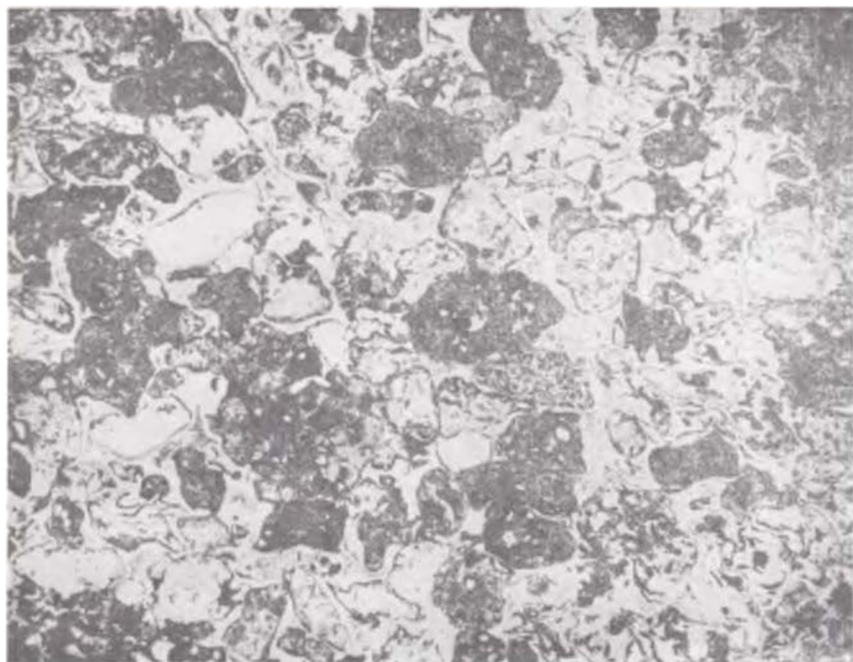
Рис. 26. Туф псаммитовый, витрокластический. Николи П., \times 28 .
