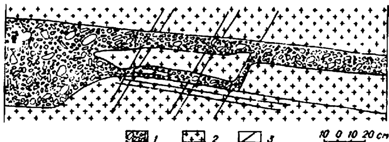
Рис. 12. Сложная брекчневая дайка. Вышковский район:
