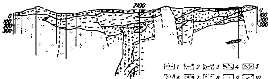
Рис. 51. Геолого-пострографический разрез по скважинам через Ильинецкую палеовулканическую структуру:
