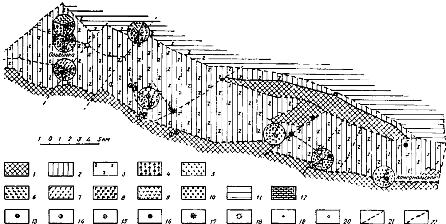
Рис. 48. Палеовулканологическая карта юго-западного Донбасса для позднедевонской эпохи.
