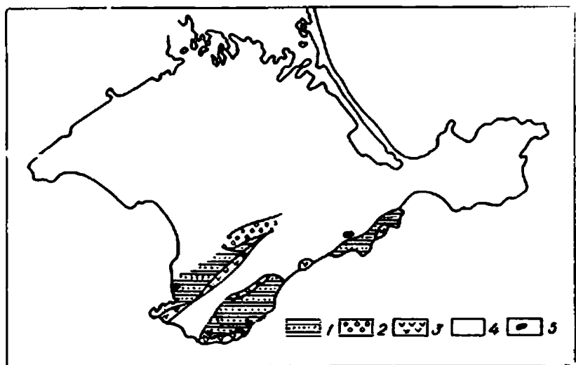
Рис. 36. Реконструкция распространения байосских отложений в Горном Крыму, по В. В. Бобылеву:
