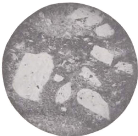
Рис. 9. Туф андезито-дацита с флюидалльной связующей массой. Чопская цепь погребенных вулканов. Сква. 15-Ч, верхний паннон. Без анализатора, \times 25 .
