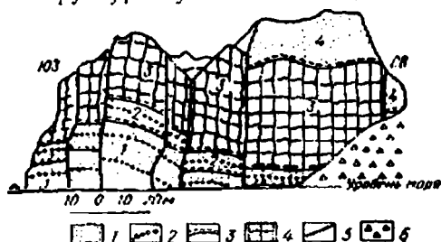
Рис. 38 Сбросы в береговых обрывах мыса Ифгени, по А. И. Шалимову (1960):
