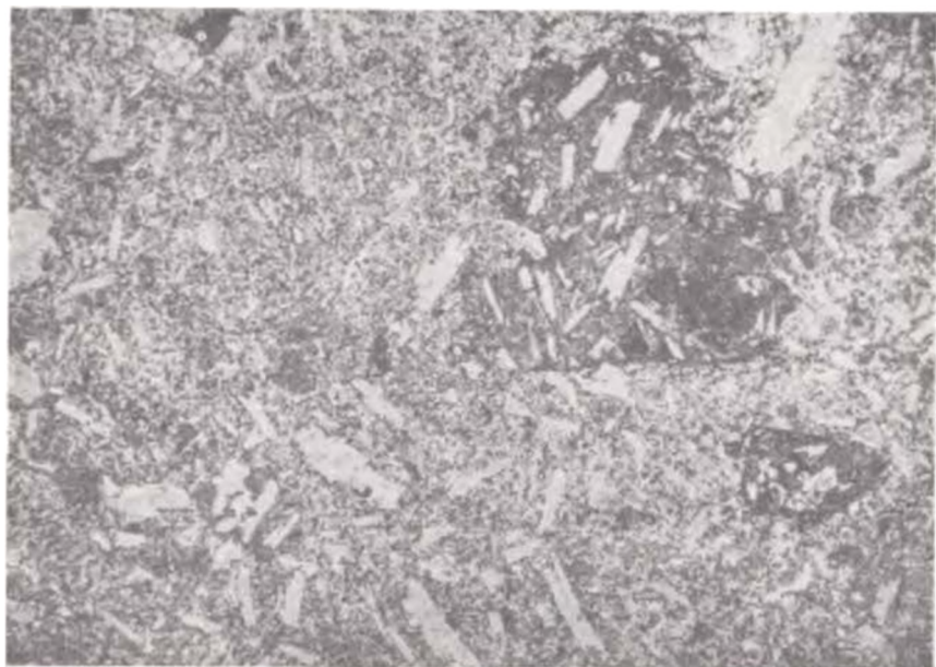
Рис. 47. Брекчиевый базальт балки Цыганки под микроскопом. Николи I, X 40
