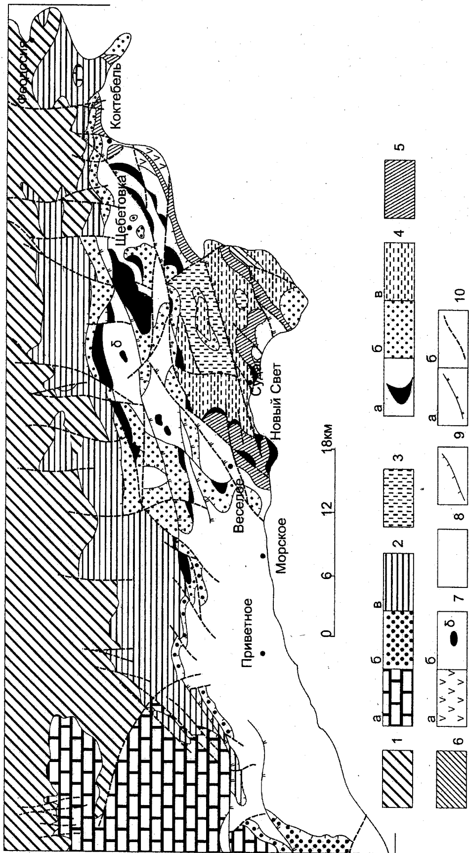
Рис. 3. Тектоническая схема Восточного (Судакского) сектора Горного Крыма (с использованием материалов геологических съемок М.В. Муратова, Г.И. Немкова и др.): 1 — меловые отложения платформенного чехла; 2—7а — дигитации, сложенные: 2 — титонско-нижнеберриасскими отложениями яйлинской серии (а — карбонатными, б — конгломератами, в — глинистыми); 3—6 — судакской серии: 3 — кимериджскими песчано-глинистыми отложениями, 4 — оксфордскими отложениями (а — известняками, б — конгломератами и песчаниками, в — глинами и песчаниками), 5 — келловейскими песчано-глинистыми отложениями, 6 — батскими песчано-глинистыми отложениями; 7а — верхнебайосскими осадочно-вулканогенными образованиями карадагской серии; 7б — среднеюрский шток диоритов; 8 — верхнетриасово-среднеюрский флиш таврической серии; 9—10 — разрывы: 9 — пологие надвиги и покровы, 10 — крутые разломы; а — продольные ластрические сбросы, б — косые и поперечные сбросы, в — сбросы и сдвиги
