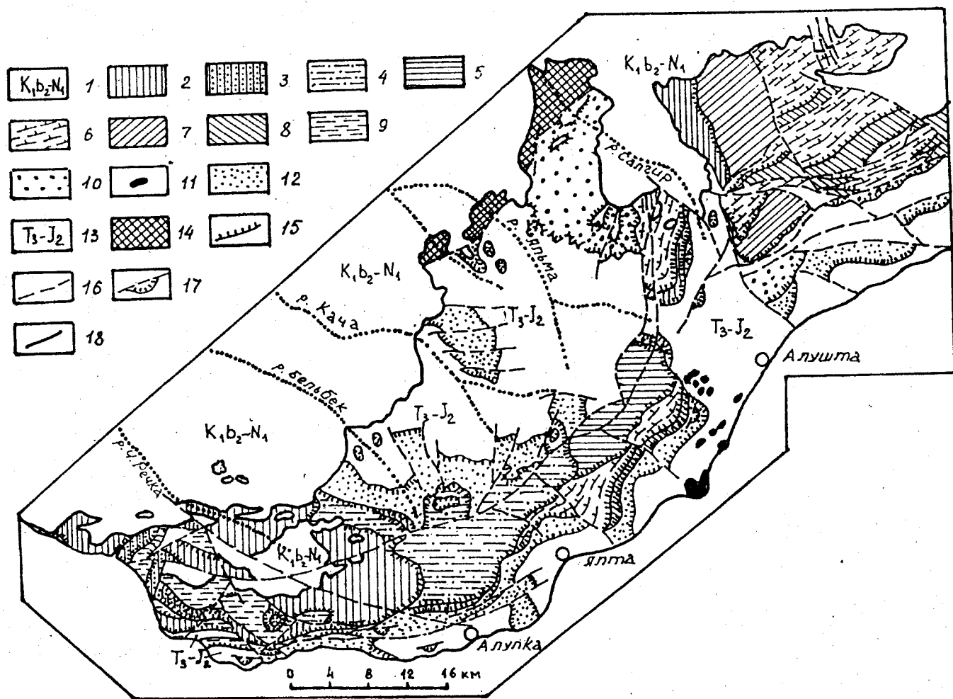
Рис. 2. Тектоническая схема дигитаций верхней структурной единицы Западного и Центрального секторов Горного Крыма: 1 — платформенный чехол Скифской плиты, представленный меловыми, палеогеновыми и миоценовыми отложениями; 2–14 — киммерийский горно-крымский структурный комплекс: 2–13 — Горно-Крымская структурная зона: 2–10 — верхняя структурная единица, представленная дигитациями, сложенными титонско-нижнеберриасскими, частично киммериджскими отложениями: 2 — карбонатными, 3 — переслаивание пудинговых известняков и конгломератов, 4 — тектоническое переслаивание (дуплексы) известняков и мергелей, 5 — мергелями, 6–8 — ритмичными карбонатно-терригенными отложениями: 6 — с преобладанием карбонатных, 7 — с преобладанием терригенных, 8 — псевдоединые карбонатные — результат тектонического сшивания карбонатных прослоев; 9–10 — преимущественно песчано-глинистыми, 10 — преимущественно песчано-конгломератовыми; 11–12 — средняя структурная единица: 11 — среднеюрские интрузивы, 12 — преимущественно образования эскиординской и карадагской серий, расчлененные и смятые в складки; 13 — нижняя структурная единица — преимущественно флиш таврической серии, расчлененный и смятый в складки; 14 — Лозовская зона смятия — мегамеланж, представленный преимущественно эскиординскими и карадагскими кластолитами и экзотическими глыбами; 15 — надвиги и покровы; 16 — взбросы, сбросы и сдвиги; 17 — тектонические отторженцы карбонатных пород; 18 — граница меловых отложений ( K_{1,b_2-N_1} )
