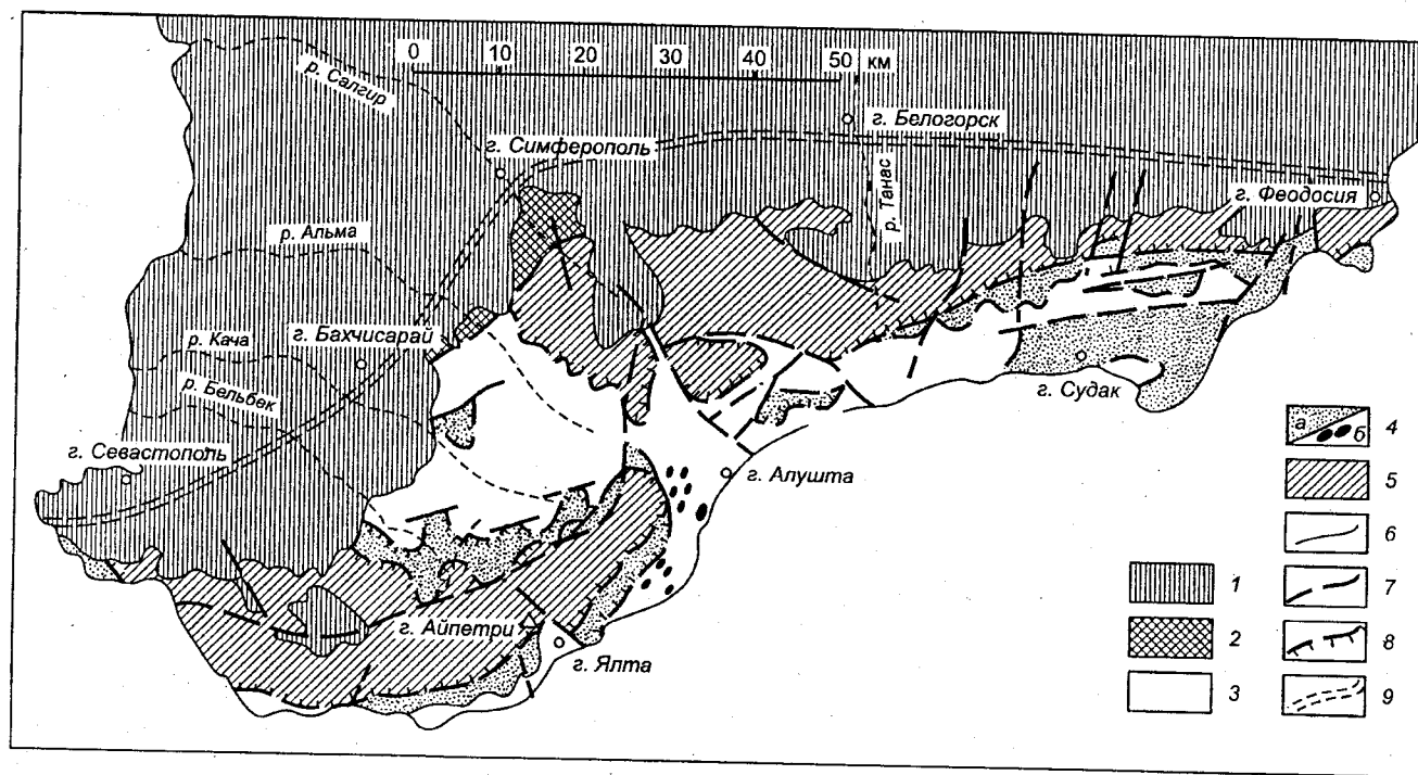
Рис. 1. Тектоническая схема Горного Крыма:
