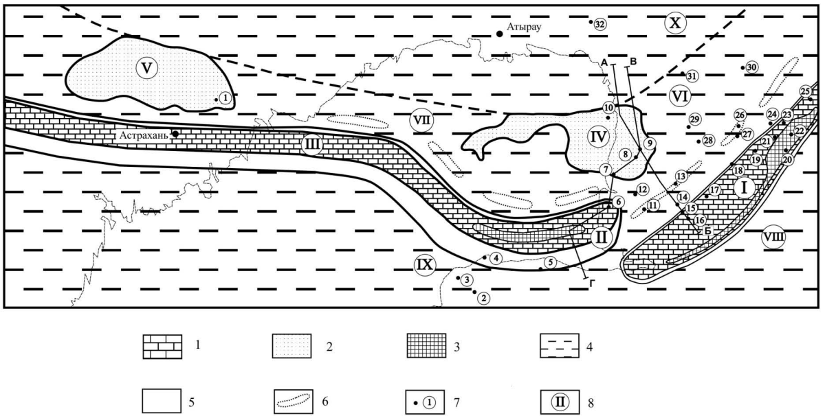
Рис.1. Карта литофаций московских отложений юго-востока Прикаспийской впадины. 1 – карбонатные отложения, 2 – переслаивание карбонатных и глинисто-карбонатных отложений, 3 – зона отсутствия осадков, 4 – преимущественно глинистые отложения, участками карбонатные отложения, 5 – переслаивание карбонатных и карбонатно-обломочных отложений, 6 – локальные палеоподнятия, 7 – скважины: 1 – 4 Имашевская, 2 – 7 Бузачи Северный, 3 – П-1 Каражанбас Северный, 4 – П-1 Арман, 5 – П-1 Каратурун Восточный, 6 – 2 Южная, 7 – 53 Тенгиз, 8 – 10 Тенгиз, 9 – 8 Королевская, 10 – П-10 Пустынный, 11 – 1 Пионерская, 12 – 10 Култук Северный, 13 – 120 Елемес, 14 – 1 Сазтубе, 15 – П-2 Сазтубе, 16 – П-1 Сазтубе Южное, 17 – 1 Бекбулат, 18 – П-2 Караой, 19 – П-1 Южно-Молодежная, 20 – П-1 Мынсуалмас Северный, 21 – 13 Южно-Эмбинская, 22 – 4 Туресай, 23 – 23 Тортай, 24 – 9 Тортай, 25 – 1 Уртатау-Сарыбулак, 26 – 3 Равнинная, 27 – 8 Равнинная, 28 – П-1 Карачунгул, 29 – П-1 Аккудук-Алахай, 30 – СГ-2 Биикжал, 31 – П-1 Тюлюс, 32 – П-3 Гурьевский свод; 8 – литолого-фациальные зоны: карбонатные платформы: I – Южно-Эмбинская, II – Южная, III – Махамбетская; затопленные карбонатные платформы: IV – Тенгиз-Кашаганская, V – Астраханская; относительно глубоководные зоны: VI – Маткен-Ушмолинская, VII – Морская; глубоководные зоны: VIII – Северо-Устьюртская, IX – Бузачинская, X – Гурьевско-Шукатская
