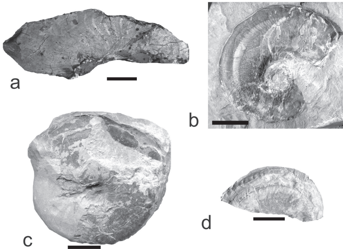
Рис.1. Кимериджские и берриасские аммониты со следами окраски (масштабная линейка 1 см): а – Neochetoceras cf. subsidens (Font.), экз. № МК2890, ГИН (сборы Рогова), Городищи (53°34'54" N; 48°25'18" E), слой 9/9, верхний кимеридж, зона Autissiodorensis , подзона Subborealis , фаунистический горизонт aff.rebholzi ; чередование светлых и темных изогнутых полос связано с схемохромией; b-c – Hyploceras ( Hypolissoceras ) cf. carachteis (Zeuschn.), мыс Ильи у г.Феодосия (45°00,827' N; 35°25,455' E), нижний берриас; b – экз. № 18/1, ЦЭНТУМ (сборы Перминова), со следами окраски в виде двух продольных полос; c – экз. № 18/2, ЦЭНТУМ (сборы Перминова), без видимых следов окраски; d – Hyploceratinae inted. , экз. № 18/2, ЦЭНТУМ (сборы Перминова), мыс Ильи у г. Феодосия (45°00,827' N; 35°25,455' E), нижний берриас; со светлой полосой в верхней части боковой стороны.
