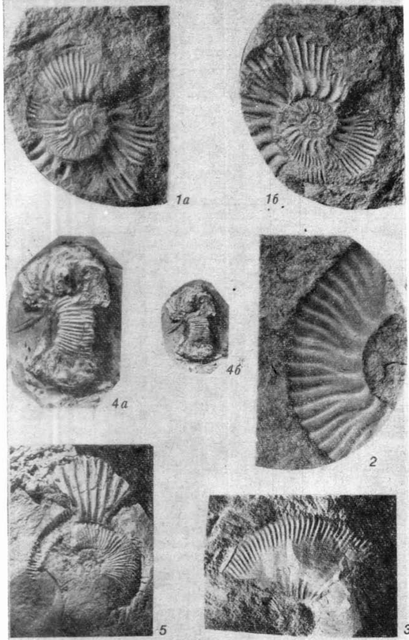
Фиг. 1, 2. Aulacostephanus ( Aulacostephanoceras ) eudoxus Ziegler; № К 11/9: а — вид с боковой стороны, б — отпечаток того же образца; Калининградская обл., Полесский р-н, скв. Ольховка-51, глубина 308,4—308,5 м; верхний кимеридж, зона eudoxus .
