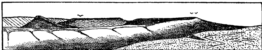
Рис. 14. Видъ внутрь Бурулькайского котла съ поверхности Петровской мулды. ~ — Бурулькая. ~ ~ — Ташлы-оба.
