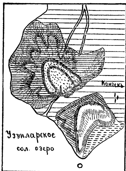
Рис. 20. Планъ горы Кончека. Широкая горизонтальная штриховка = поверхностнымъ отложеніямъ, узкая горизонтальная = M_2a , точки = M_2b , косая штриховка = M_3a , бѣлое = M_3b , черточки = руднымъ слоямъ.
