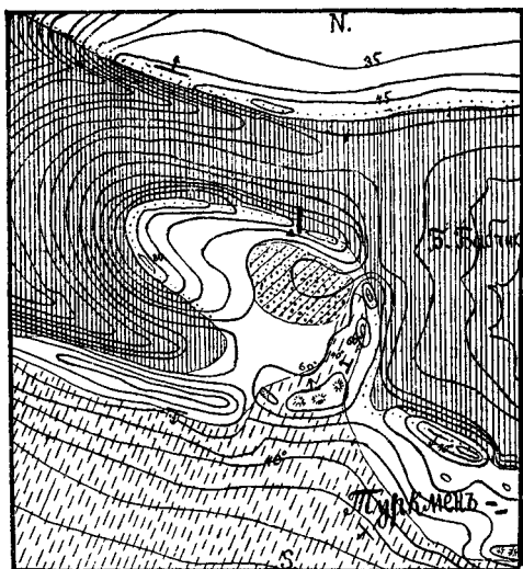
Рис. 8. Геологическая карта Бурашской котловины. Горизонтальная штриховка = M_3a , бѣлая пространства = M_3bcd , мшанковый известнякъ въ видѣ изолированныхъ горокъ, косая прерывистая штриховка — строительный известнякъ (MP), точки съ косою штриховкой — понтичскіе пласты. Маленькій треугольникъ — сѣрный ключъ, толстая черная черта — сдвигъ.
