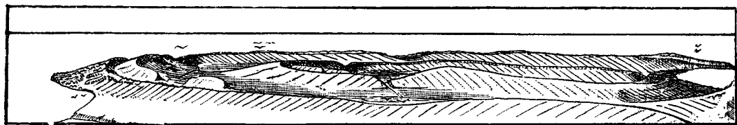
Рис. 4. Видъ профиль на Караларскую антиклиналь. ~ — гора Кичикине-чобанъ ~ ~ — Чегене, ~ — Мисырѣ, ~ ~ ~ — Джайлау, ~ ~ ~ — Сююрташъ. Внутри кольце-образный гребень чокракскаго известняка. Гора Кичикине-чобанъ — сарматскій известнякъ.
