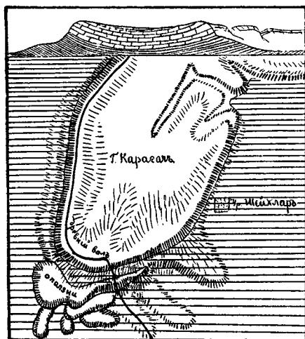
Рис. 1. Гора Карагачъ (примѣръ синклинальнаго плато). Планъ и разрѣзъ. Вверху чокракскій известнякъ (на планѣ не заштриховано), внизу темныя сланцевыя глины (горизонтальная штриховка).
