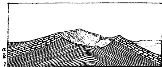
Рис. 18. Поперечный разрѣзъ Тоганашской котловины.
