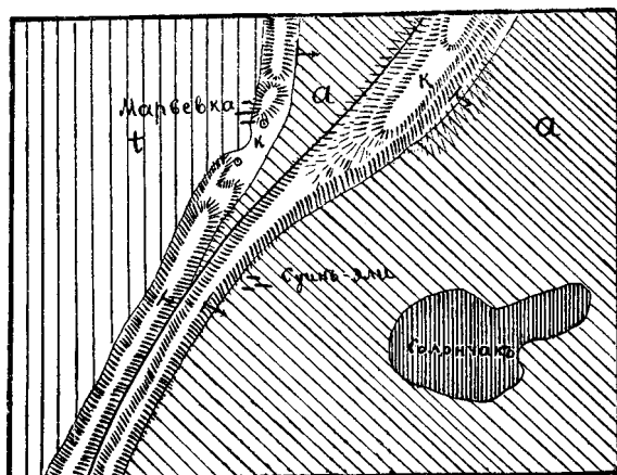
Рис. 2. Сдвигъ въ параболическомъ гребнѣ у Марьевки. a — верхнія сланцевыя глины, k — спаніодонтовые пласты и чокракскій известнякъ, t — нижнія сланцевыя глины. Толстая черта — линия сдвига.
