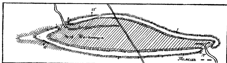
Рис. 17. Планъ Тоганапшскаго эллиптическаго гребня. Косая штрифка — M_2a , гребень — M_2bc , остальное бѣлое пространство — M_3a .
