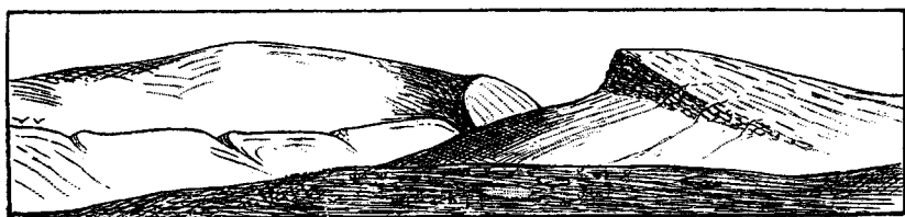
Рис. 11. Видъ на Джеултукъ (гора въ верхнемъ лѣвомъ углу— M_2a ). Направо гребень сарматскаго известняка ( M_3b ), по срединѣ гряда чокракскаго известняка — ( M_2b ).
