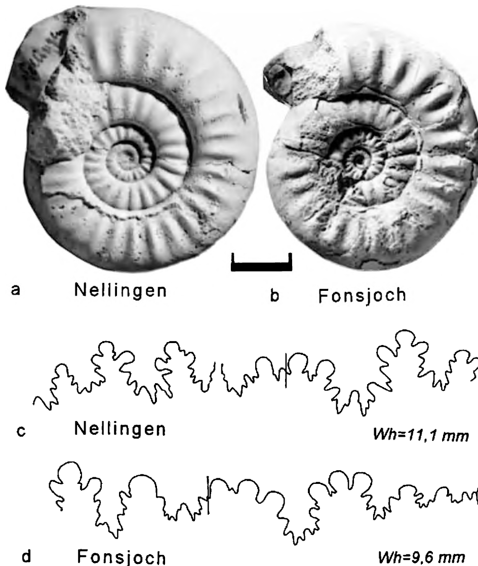
Fig. 8. Psiloceras plicatulum , NW-European and Mediterranean. Scale 1 cm. a: SMNS 64866; b: SMNS 64865; c: SMNS 64866; d: SMNS 64865.
