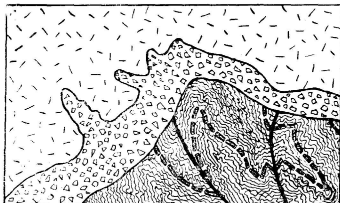
Рис. 1. Зарисовка контакта подошвы конического биогерма (гора Сахарная Голова в окрестностях г. Судака) со складчатым цоколем
