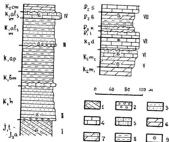
Рис. 2. Стратиграфический разрез мезозойских и кайнозойских отложений окрестностей Бахчисарая и положение в нем остатков десятиногих ракообразных:
