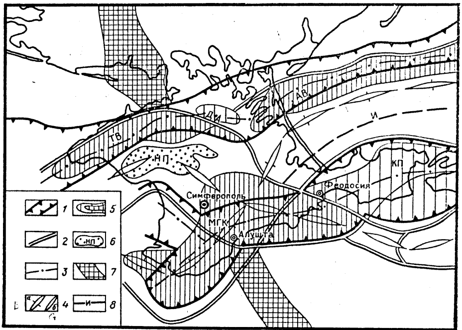
Рис. 2. Схема соотношения раннекимерийских прогибов, структур доверхнепалеозойского основания и альпийских поднятий, возникших на месте раннекимерийских прогибов
