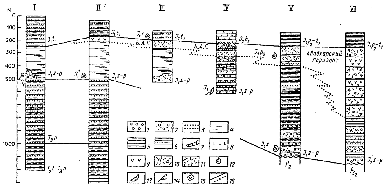
Рис. 2. Стратиграфические разрезы триасовых и нижнеюрских отложений Лозовской зоны Крыма и Псеашхинской зоны Северо-Западного Кавказа: I — вторая тектоническая чешуя, II — первая тектоническая чешуя, III — аллохтонная пластина севернее горы Астроблема, IV — долина р. Салгир, V — р. Авадхара, VI — пер. Санчаро; 1 — конгломераты; 2 — крупнозернистые кварцевые песчаники, гравелиты и конгломераты; 3 — мелкозернистые песчаники; 4 — алевролиты; 5 — аргиллиты; 6 — тонкоритмичный флишиод; 7 — известняки; 8 — лавы микродиабазов, спилитов; 9 — лавы андезитов; 10 — туфы, туфобрекчии андезитового состава; 11 — туфы, туфобрекчии кислого состава; 12 — находки аммонитов; 13 — брахиоподы; 14 — находки древесины; 15 — спорово-пыльцевые комплексы; 16 — границы свит (а) и фациальные границы (б); Б.А.Г. — бодрак-альминский вулканогенный горизонт
