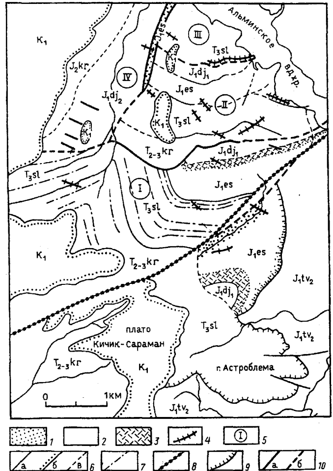
Рис. 1. Геологическая карта участка Бодрак-Альминского водораздела: 1 — грубообломочная фация; 2 — глинисто-алевритовая фация; 3 — вулканогенная фация; 4 — верхнебайосские дайки андезитов, андезито-базальтов, долеритов; 5 — номера тектонических чешуй в Лозовской зоне; 6 — стратиграфические границы (а — согласные, б — несогласные, в — предполагаемые); 7 — маркирующие горизонты, отдешифрованные по АФС; 8 — Бодракский разлом; 9 — надвиги в основании аллохтонных пластин; 10 — прочие разрывные нарушения (а — достоверные, б — предполагаемые); K_1 — нижнемеловые отложения, J_2kr — карагачская свита, J_1dj_2 — верхнеджидаирская подсвита, J_1dj_1 — нижнеджидаирская подсвита, J_1tv_2 — верхнетаврическая свита, J_1es — эскиординская свита, T_3sl — салгирская свита, T_2-3kr — курцовская свита
