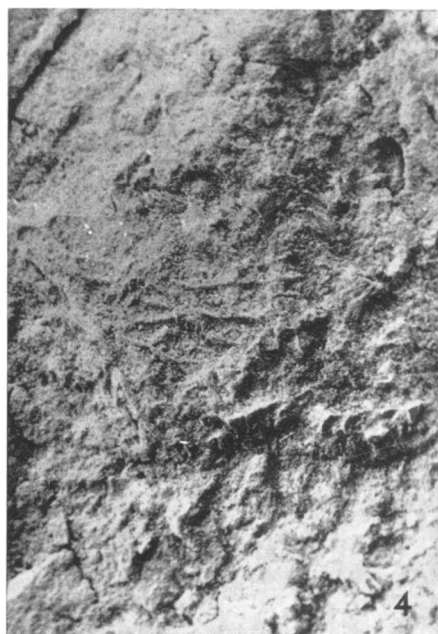
Abb. 4—5. Oberflächendetail einer Lumbricaria . Solnhofener Plattenkalke, Unter-tithon, Schernfeld. 1964 XXIII 107; Stereoscan-Aufnahmen.
