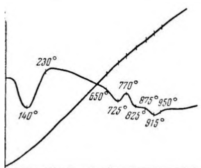
Рис. 4. Кривая нагревания фракции (уд. в. 2,47—1,80) оглановитического бентонита
