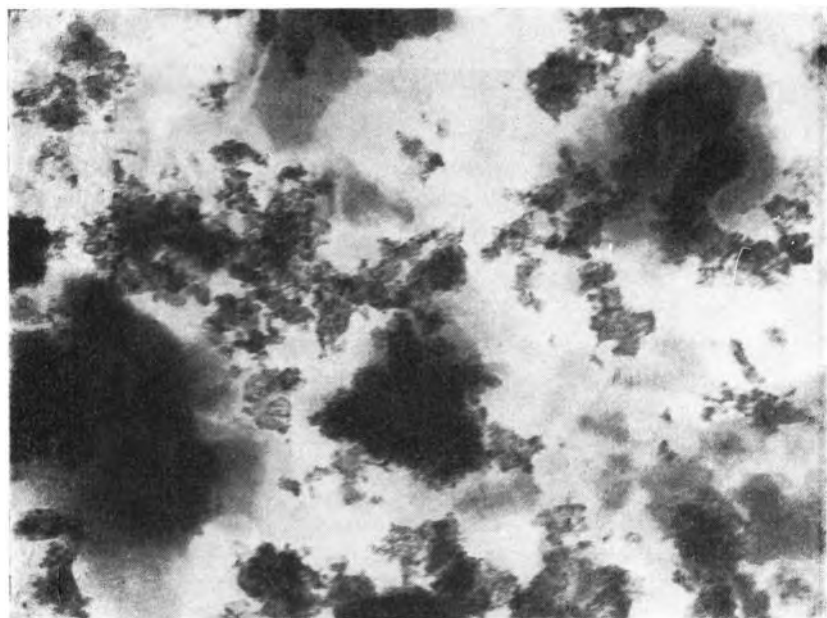
Рис. 6. Электронномикроскопическая фотография фракции (уд. в. 2,47—1,80) отгланцированного бентонита ( \times 12\,000 )
