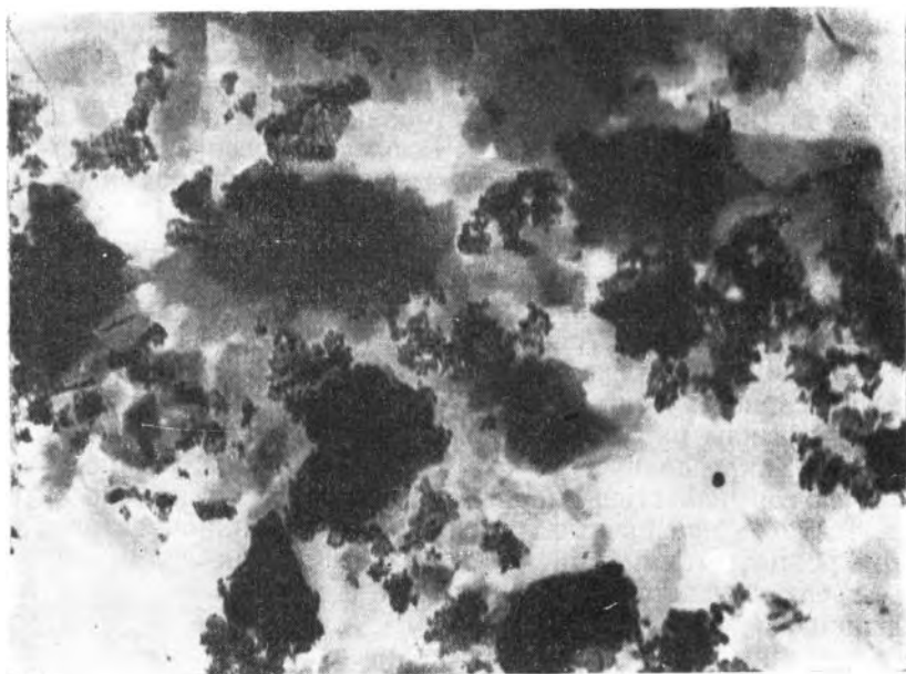
Рис. 8. Электронномикроскопическая фотография фракции (уд. в. <1,80) оглялинского бентонита ( \times 12\,000 )
