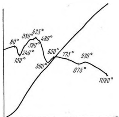
Рис. 68. Кривая нагревания. Омск, скв. I-Р, глубина 857—863 м
