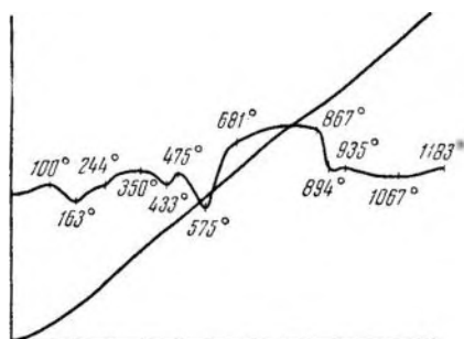
Рис. 36. Кривая нагревания. Ханты-Мансийск, скв. I-Р, глубина 1999,26—2011,9 м
