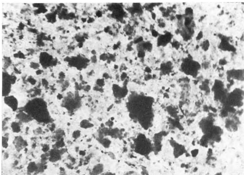
Рис. 63. Электронномикроскопическая фотография. Омск, скв. I-Р, глубина 1923—1929 м ( \times 12\,000 )
