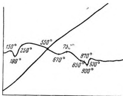
Рис. 11. Кривая нагрева фракции (уд. в. 2,47—1,80) гилляби
