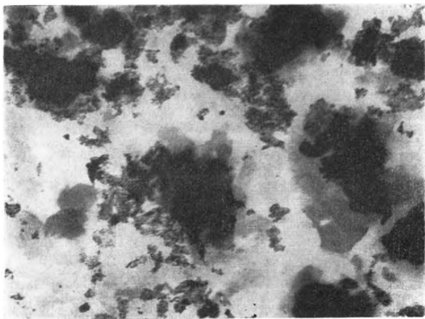
Рис. 7. Электронномикроскопическая фотография фракции (уд. в. 2,47—1,80) оглялинского бентонита ( \times 12\,000 )
