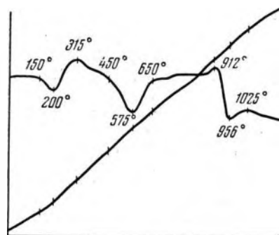
Рис. 18. Кривая нагревания коллоидной фракции, полученной методом отстаивания. Березово, скв. 1-Р, глубина 1245—1251 м
