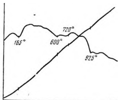
Рис. 12. Кривая нагрева фракции (уд. в. <1,80) гилляби
