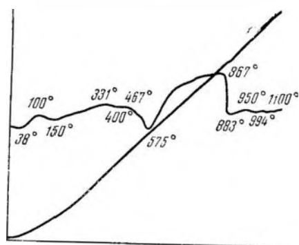
Рис. 37. Кривая нагревания. Ханты-Мансийск, скв. I-Р, глубина 1929,33—1935,63 м
