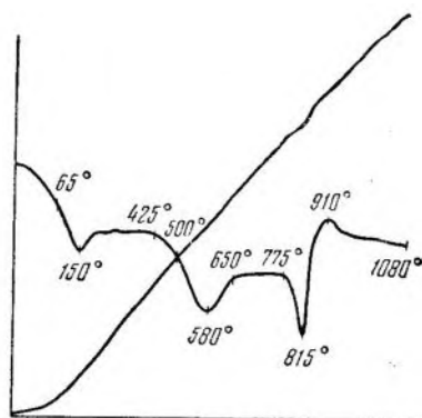
Рис. 60. Кривая нагревания. Омск скв. I-P, глубина, 2289,8—2283,8 м
