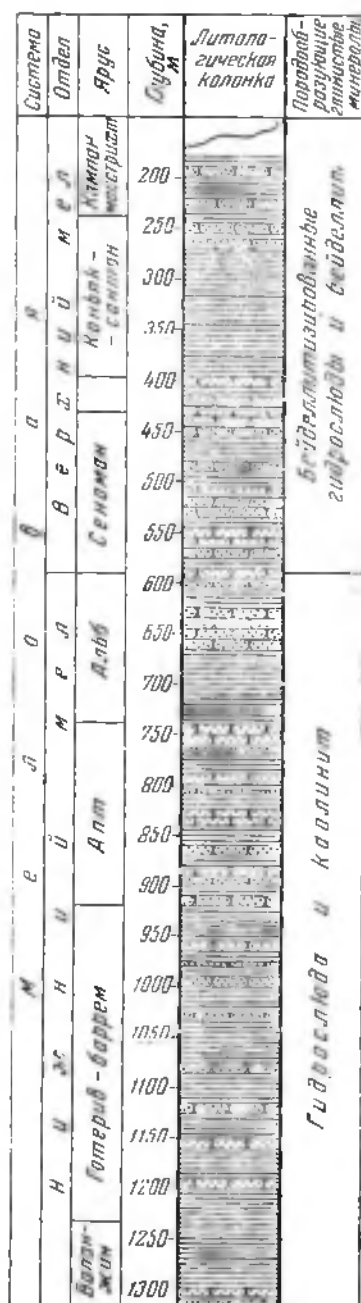
Рис. 20. Разрез скв. 1-Р, Берзово: 1 — глины; 2 — песчано-александровые породы
