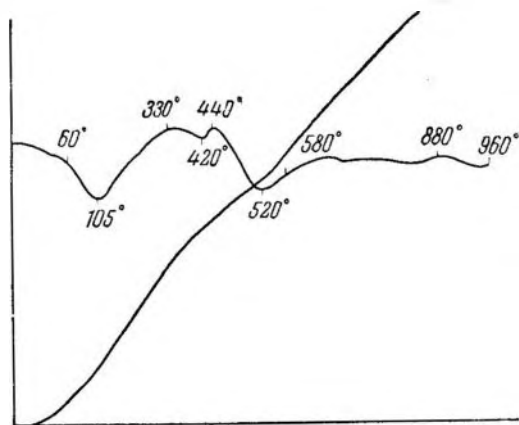
Рис. 28. Кривая нагревания. Березово, скв. I-Р, глубина 227—228 м
