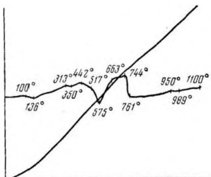
Рис. 39. Кривая нагревания. Ханты-Мансийск, скв. I-Р, глубина 1665,65—1673,40 м
