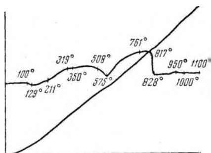
Рис. 38. Кривая нагревания. Ханты-Мансийск, скв. I-Р, глубина 1722,9—1730,9 м
