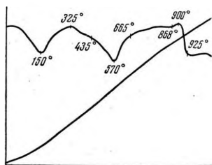
Рис. 19. Кривая нагревания коллоидной фракции, выделенной на центрифуге и осажденной электролитом. Березово, скв. 1-Р, глубина 1245—1251 м
