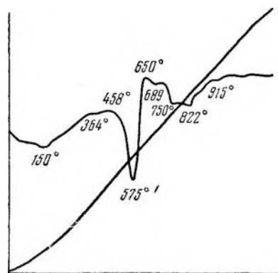
Рис. 59. Кривая нагревания. Омск скв. I-P, глубина 1923—1929 м
