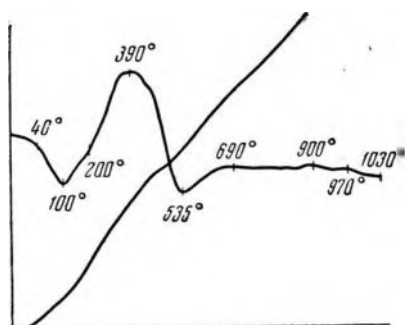
Рис. 16. Кривая нагрева породы Березово, скв. 1-Р, глубина 1245—1251 м
