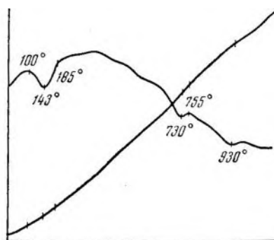
Рис. 5. Кривая нагревания фракции (уд. в. <1,80) оглановитического бентонита
