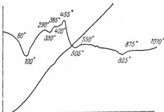
Рис. 29. Кривая нагревания. Березово, скв. 1-Р, глубина 273—275 м
