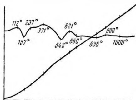
Рис. 49. Кривая нагревания. Ханты-Мансийск, скв. 1-Р, глубина 842,55—854,5 м
