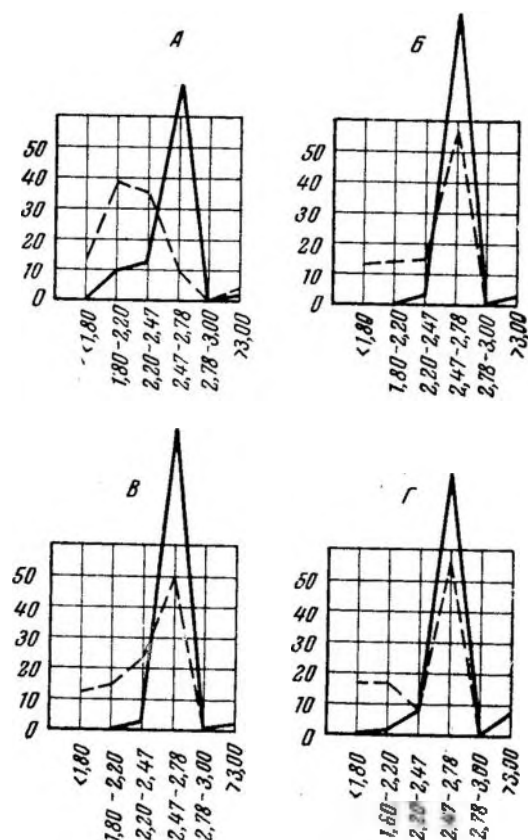
Рис. 30. Кривые гравитационного анализа. Березово, скв. I-P:
