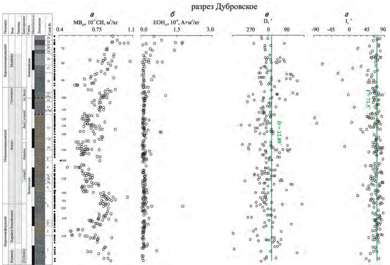
Рис. 4. Разрез Дубровское: а — величина удельной магнитной восприимчивости, б — величина удельной естественной остаточной намагниченности, в — склонение характеристической компоненты намагниченности, г — наклонение характеристической компоненты намагниченности. Зеленым показаны современные значения склонения и наклонения. Условные обозначения см. рис. 3
