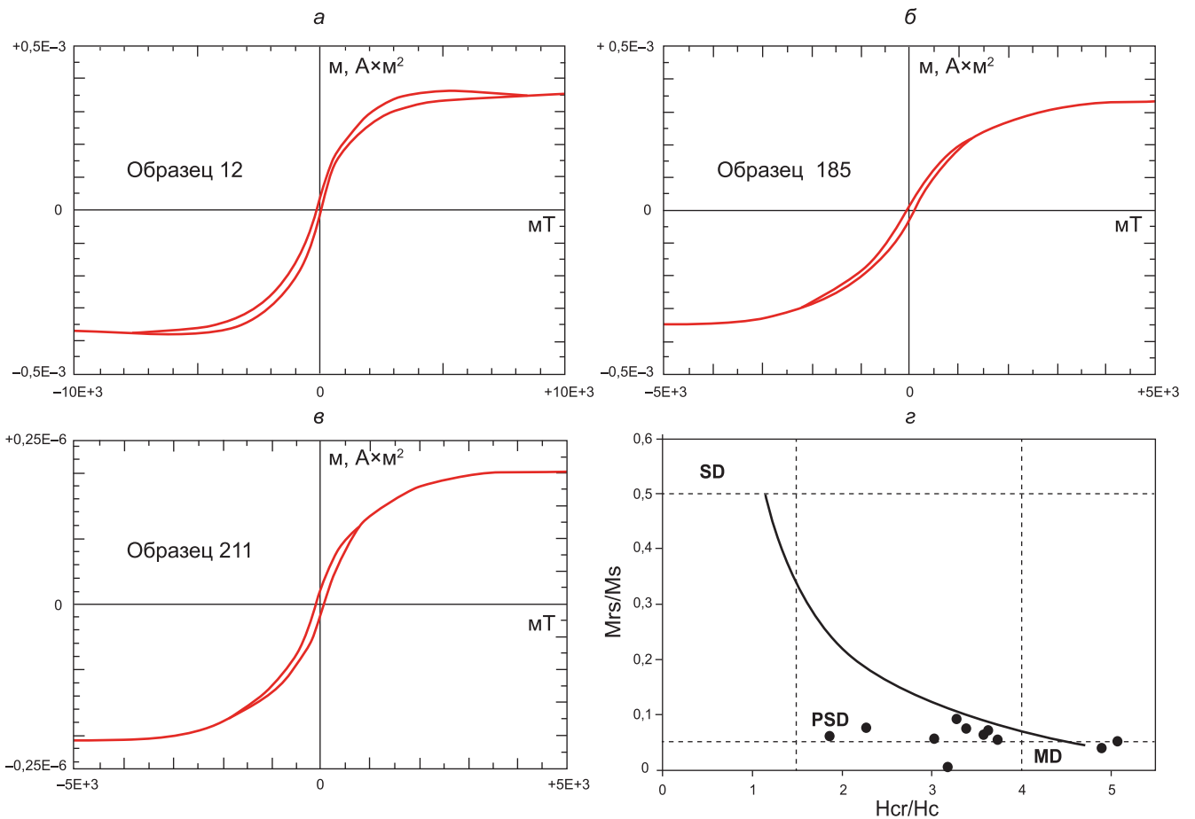
Рис. 7. Петли гистерезиса после удаления пара- и диамагнитного вкладов (а–в) и диаграмма Дэй (г) [Day, et al., 1977]. Ms — намагниченность насыщения, Mrs — остаточная намагниченность насыщения, Hc — коэрцитивная сила, Hcr — остаточная коэрцитивная сила, SD — однодоменные частицы, PSD — псевдооднодоменные частицы, MD — многодоменные частицы
