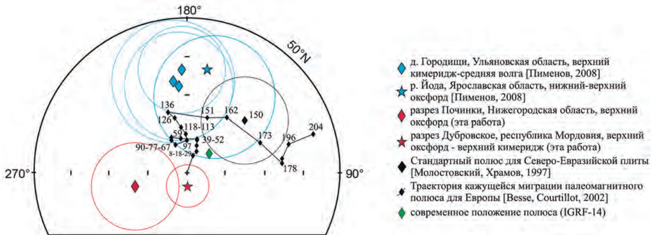
Рис. 12. Сравнение палеомагнитных полюсов, полученных по верхнеюрским отложениям Русской плиты, с кривой кажущейся миграции палеомагнитного полюса Восточно-Европейской платформы [Besse, Courtillot, 2002] (числами показаны возрасты полюсов)
