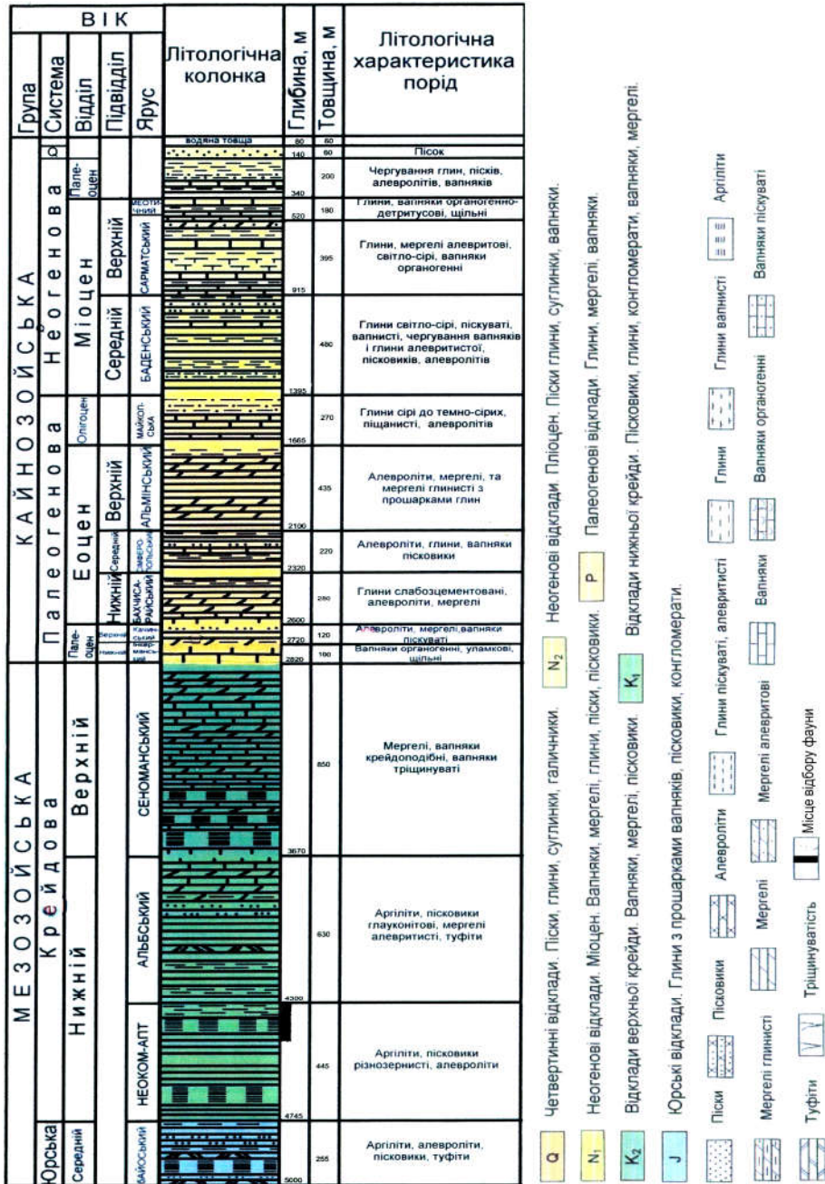
Розріз свердловини Степова-І.
