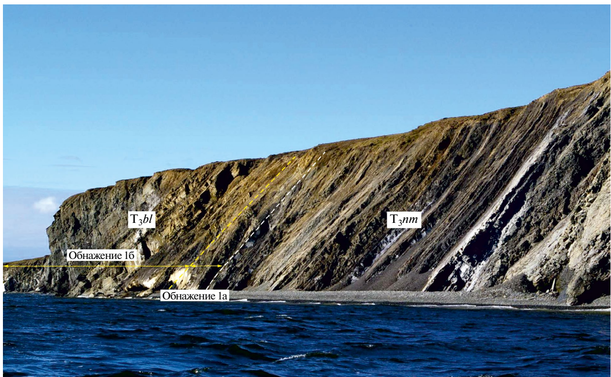
Рис. 3. Общий вид обнажений 1а и 1б. Желтая пунктирная линия — граница свит. Фото Н.Н. Соболева (2007 г.)
