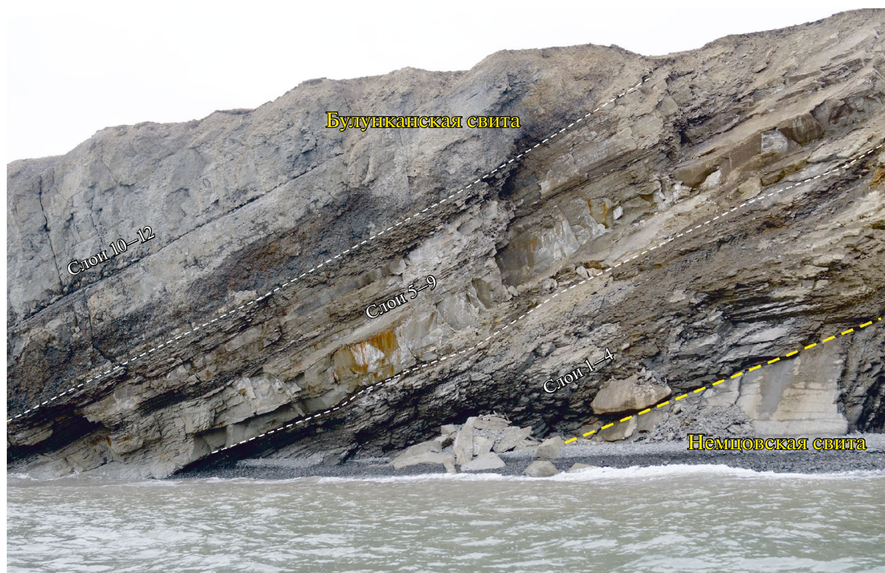
Рис. 5. Контакт немцовой и булунканской свит на мысе Конгломератовый. Желтая пунктирная линия — граница свит. Белые пунктирные линии — границы слоев. Фото А.Ю. Попова, 2014 г.
