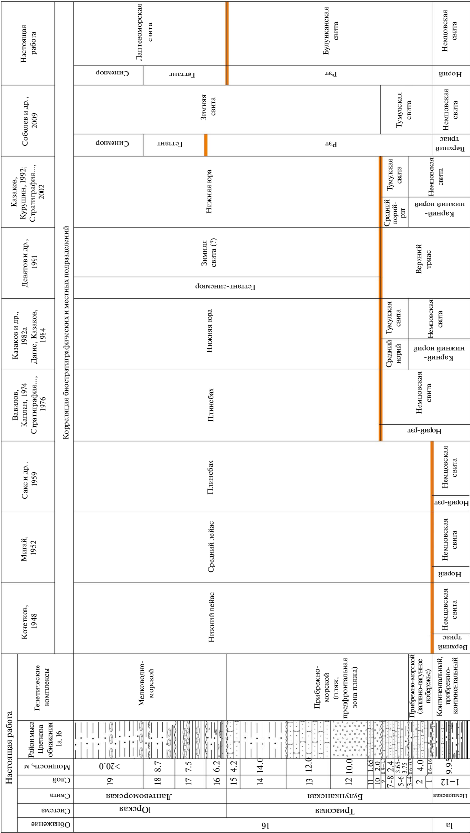
Рис. 2. Ретроспектива взглядов на положение границ биостратиграфических и местных подразделений в пограничных отложениях триаса и юры в районе мыса Цветкова. Красная линия – граница триаса и юры; сплошные горизонтальные линии – границы свит. Условные обозначения см. на рис. 4
