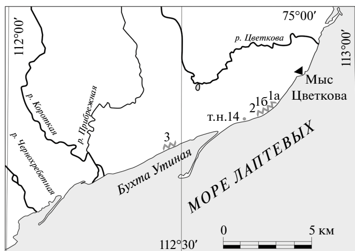
Рис. 1. Карта-схема расположения изученных обнажений на западном берегу Хатангского залива
