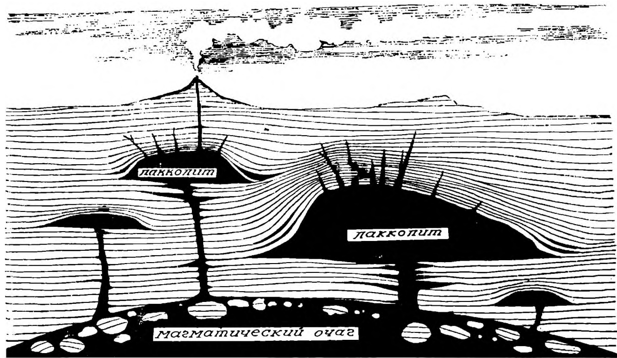
Рис. 3. Лакколиты.
