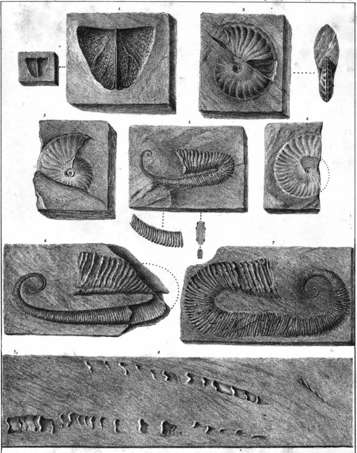
1. Trigonellites radians Giebel ( Crétacé ). - 2-4. Ammonites Masylaeus Coquand ( Crétacé ). - 5-7. Ancyloceras Sabaudianum Pictet et de Loriol ( Crétacé ). - 8. Baculites Meyrati Ooster ( Crétacé ).
