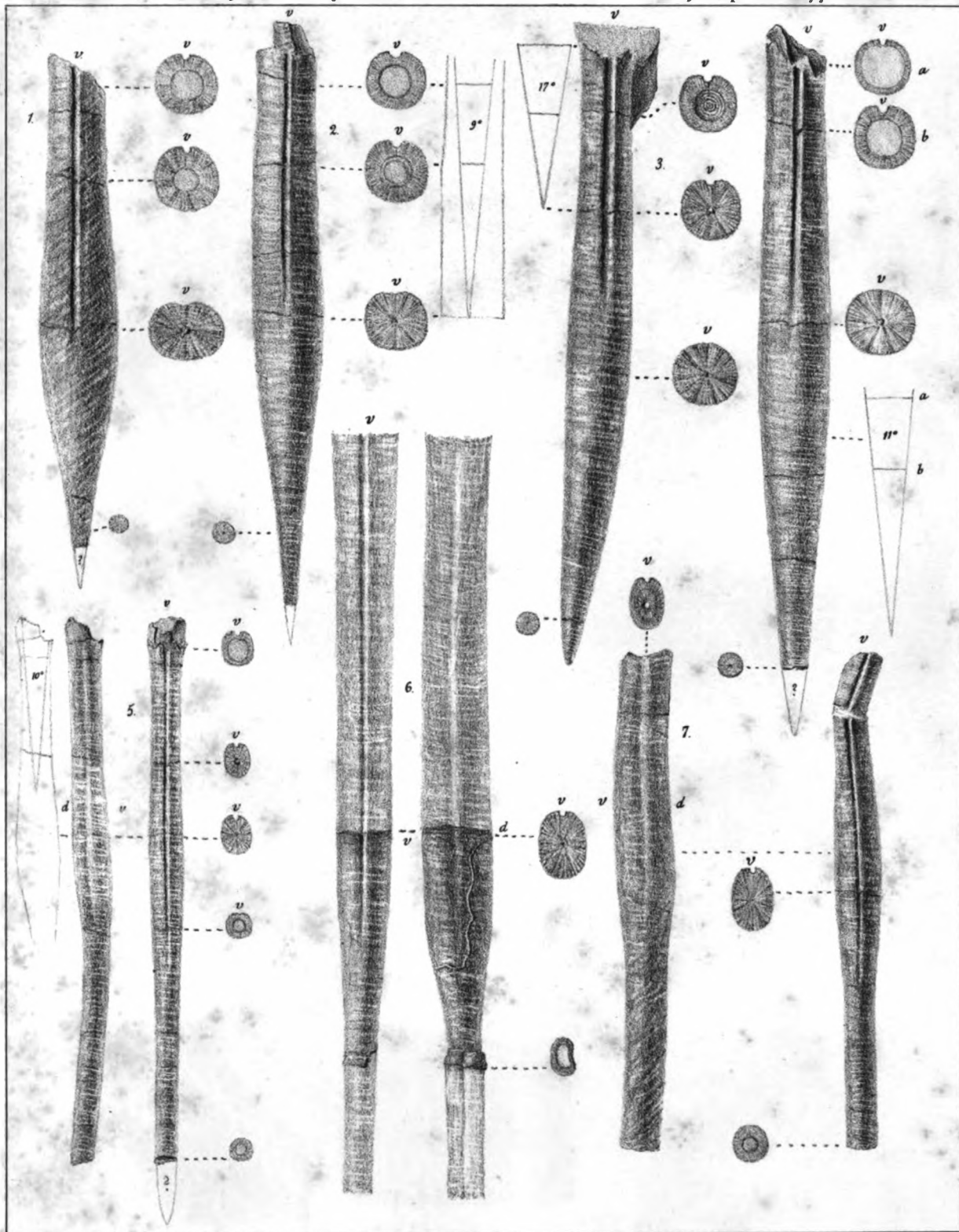
1-4. Belemnites semicanaliculatus Blainville, variétés ? (Crétacé). - 5-7. Belemnites Lorioli Ooster (Crétacé). -
