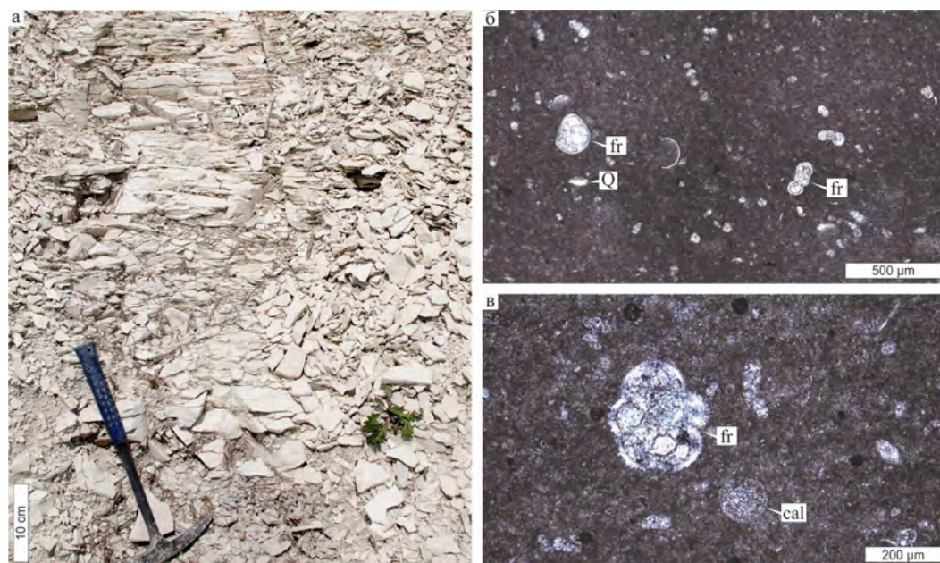
Рис. 5. ЛТ3 – известняки, вакстоуны мендерской свиты, г. Кременная: а – в обнажении, б, в – в шлифах (б – николи II, в – николи X). Q – кварц, fr – фораминиферы, cal – кальцисферы.
