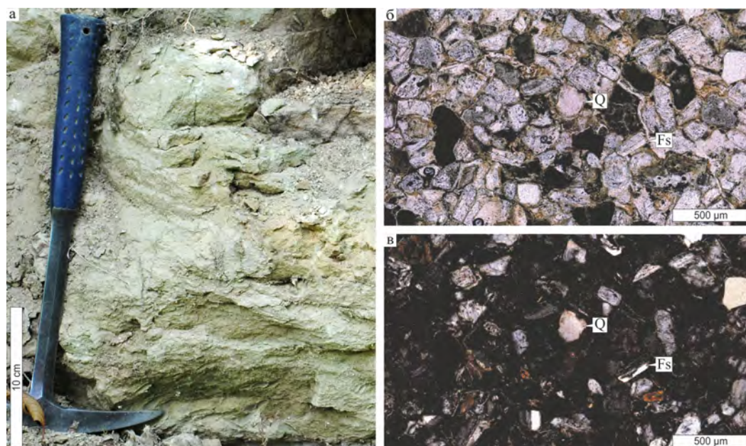
Рис. 8. ЛТ6 – песчаники белогорской свиты, р. Бодрак: а – в обнажении, б, в – в шлифе (б – николи II, в – николи X). Q – кварц, Fs – полевоы шпат.
