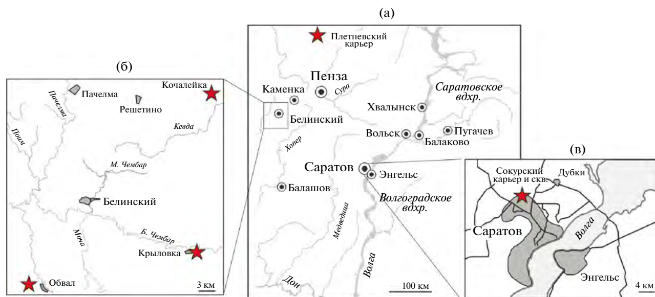
Рис. 4. Расположение разрезов (отмечены звездочками) (по Тесакова, 2022г, с дополнениями).
