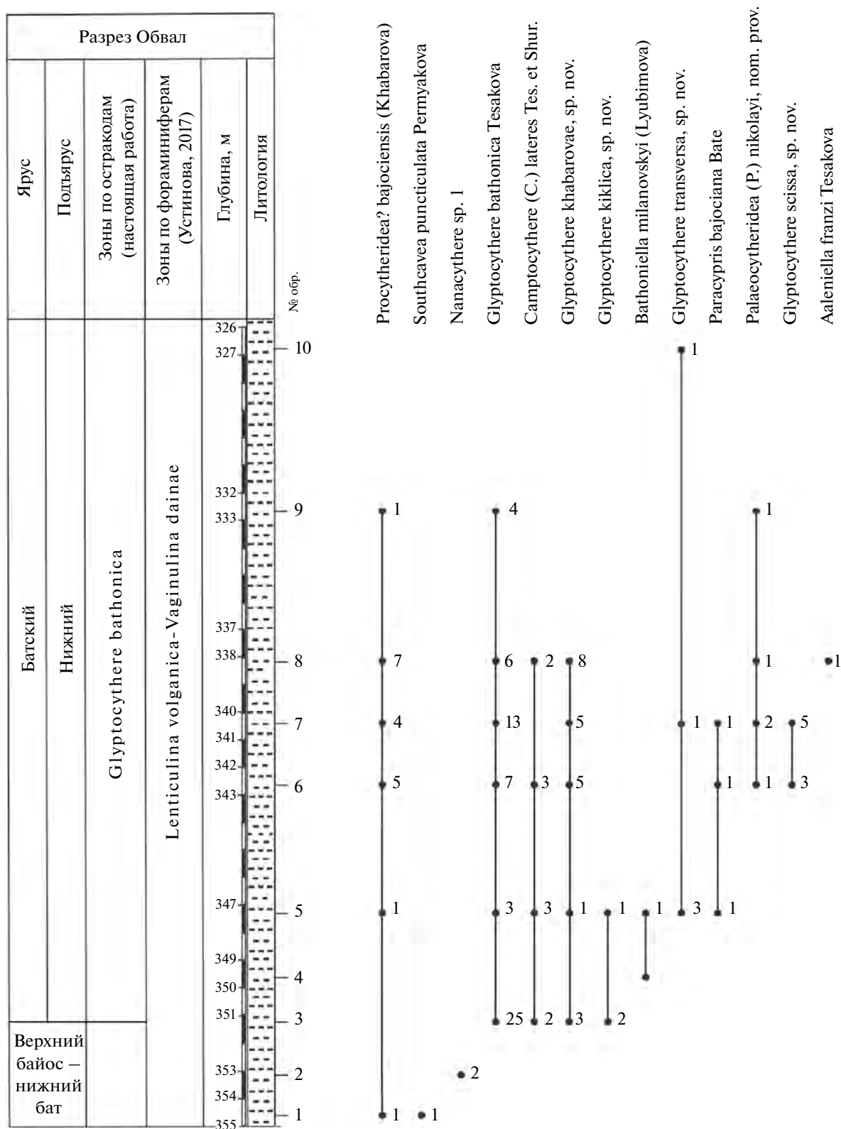
Рис. 8. Распространение остракод по разрезу скв. Обвал, Тамалинский р-н, Пензенская обл.
