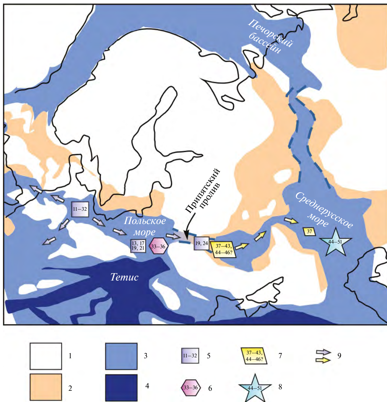
Рис. 2. Распространение остракод рода Glyptocythere в Центральной и Восточной Европе. Палеогеографическая карта для раннебатоцкого века (из Ипполитов, 2018, рис. 5, с изменениями).
