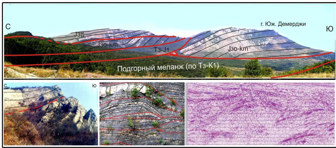
Рис. 8. Эндогенно-тектонические несогласия в обнажениях Крыма и в сейсмическом разрезе
