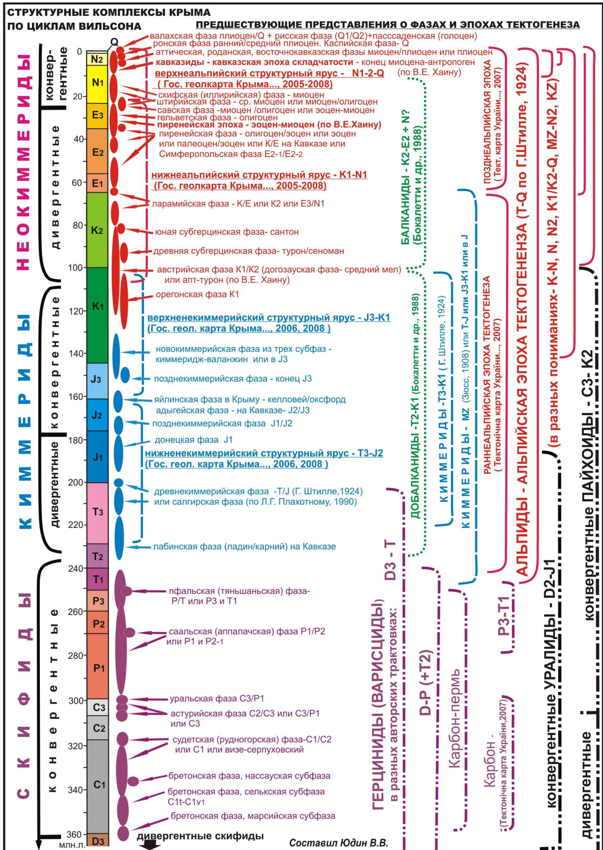
Рис. 3. Структурно-геодинамические комплексы Крыма и фазы тектогенеза Европы
