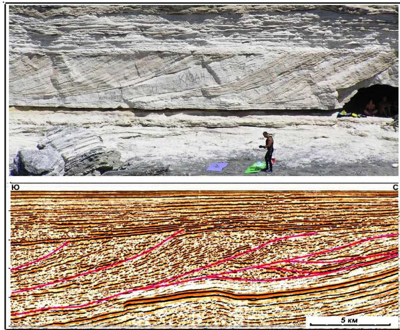
Рис. 7. Проградационные несогласия: в обнажении на мысе Атлеш (вверху) и осложненный надвигами аналог на сейсмопрофиле северо-западного шельфа Черного моря (внизу)
