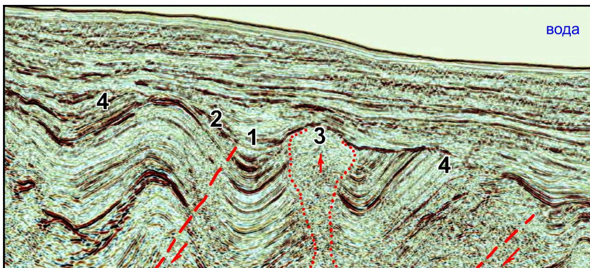
Рис. 1. Разные типы несогласий на морском сейсмопрофиле: 1- субсогласное в синклиналиях, 2- прилегания на крыльях, 3- облекания в сводах, 4- угловые несогласие
